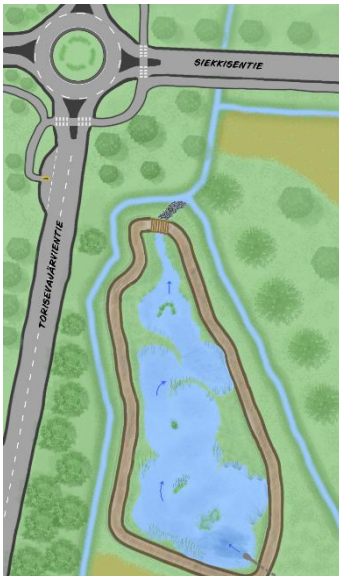
Havainnekuva kosteikosta
